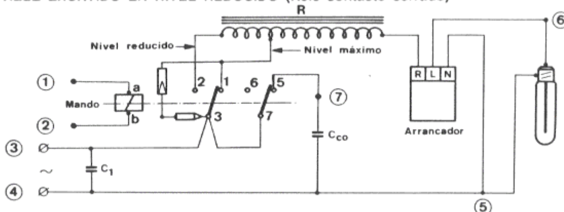
RELE EXCITADO EN NIVEL REDUCIDO (Relé contacto cerrado)
